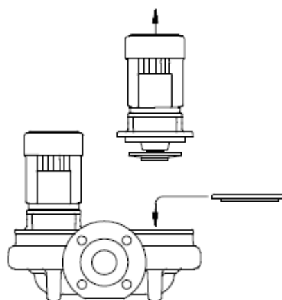
Fig. 4 Установка глухого фланца
